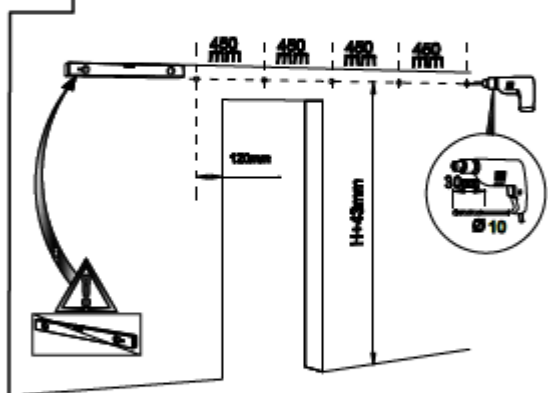
2A Montage op muur van steen / beton - Wand aus Stein / beton Stone / concrete wall - Mur à briques / béton
