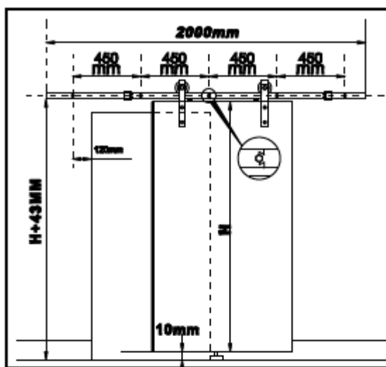
1A Montage op muur van steen / beton - Wand aus Stein / beton Stone / concrete wall - Mur à briques / béton
